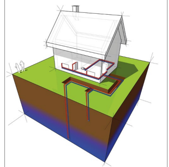
MODELL EINER GRUNDWASSER- WÄRMEPUMPE
